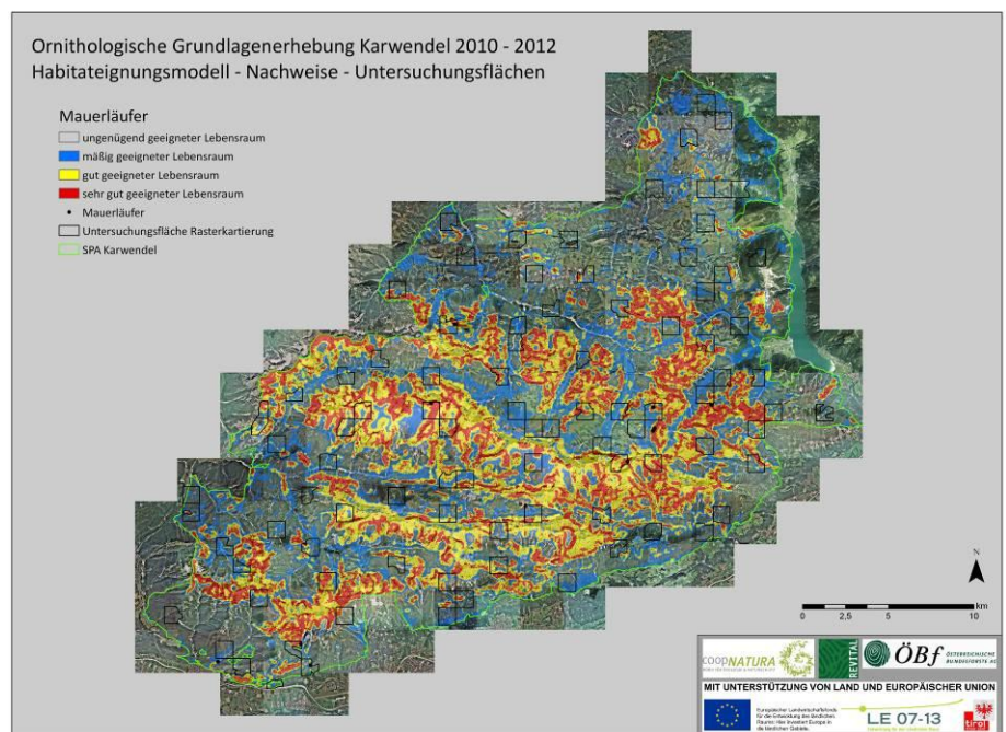
Abbildung 35: Mauerläufer – Habitateignung, Nachweise, Untersuchungsflächen
